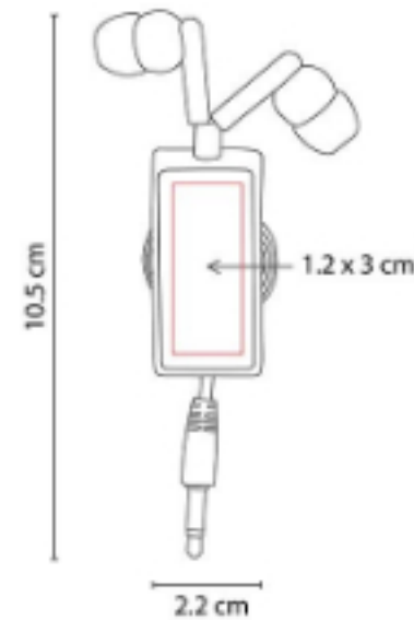
Audífonos retráctiles con clip. Miden 90 cm extendidos aproximadamente.
